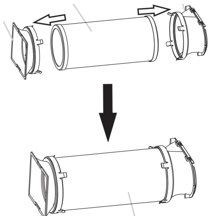
montaje de la manguera de escape
